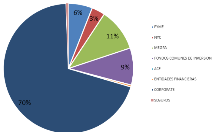
BackTest
