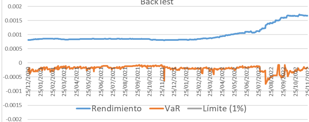
BackTest
